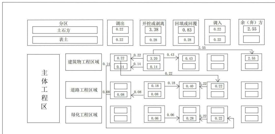
图 2-1 土石方流向图 单位：万 m 3
