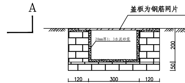
排水沟剖面图 1: 100
