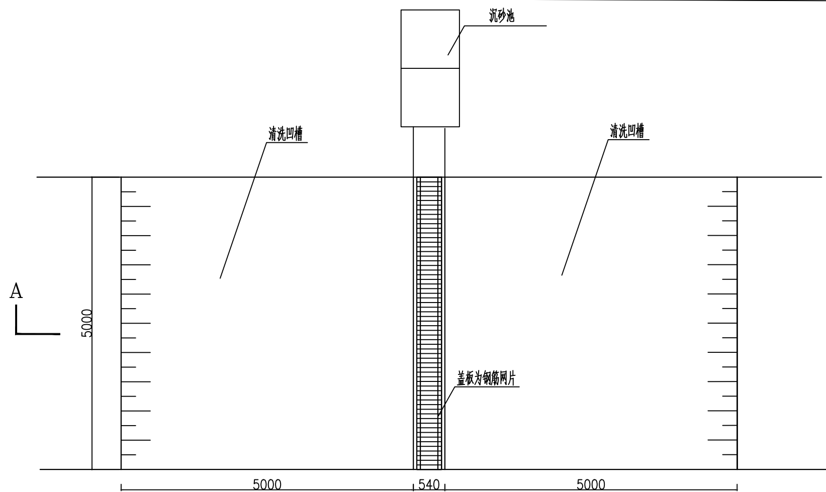
清洗槽平面图 1: 100
